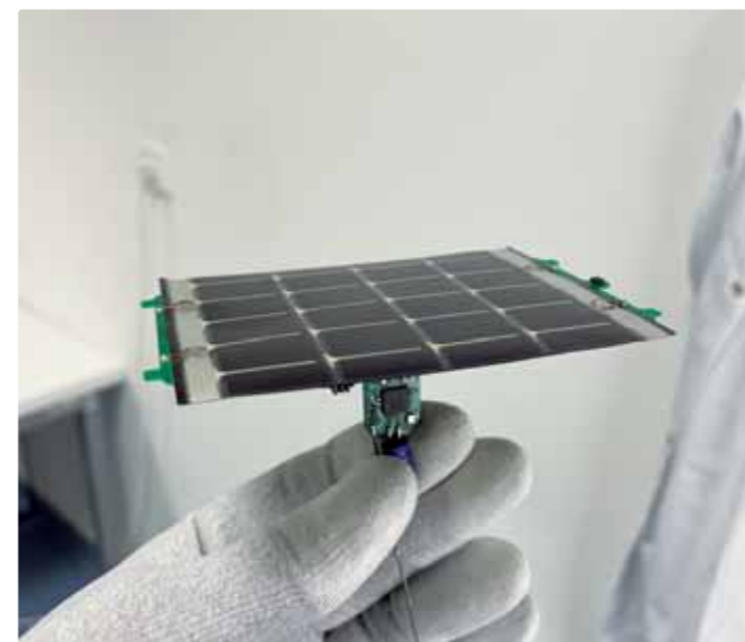
Sonda so slnečným kolektorom pre pikobalón
